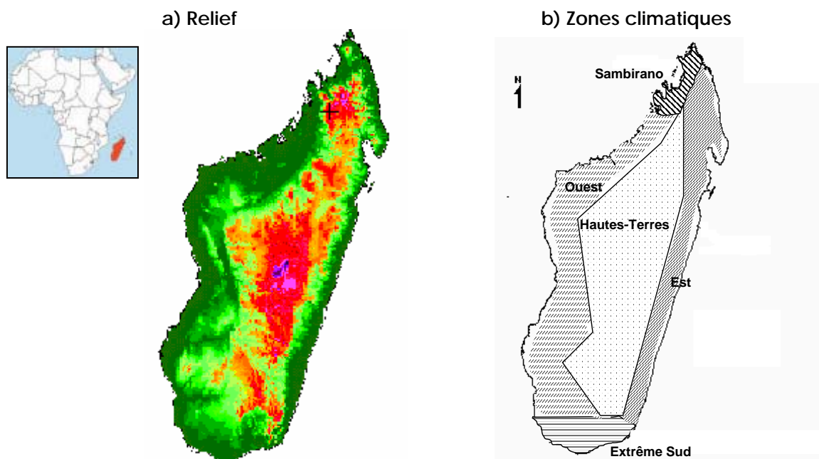
Figure 0-1 : Cartes du relief et des différentes zones climatiques, Madagascar.
