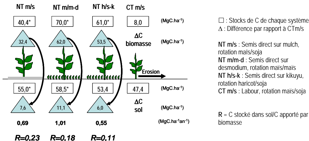
Figure 5-1 : Bilan de C sur 0-20 cm sur les systèmes en SCV et en labour conventionnel du dispositif d'Andranomanelatra.
