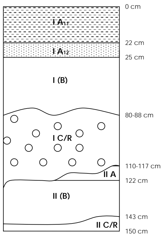
Figure 2-2 : Profil pédologique du sol. Andranomanelatra, Madagascar.
