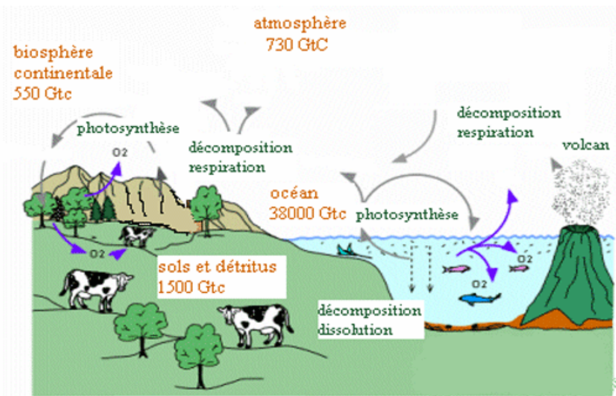
Le cycle du carbone ( http://www.cnrs.fr/cw/dossiers/dosclim/motscles/Images/cycleC.html )
