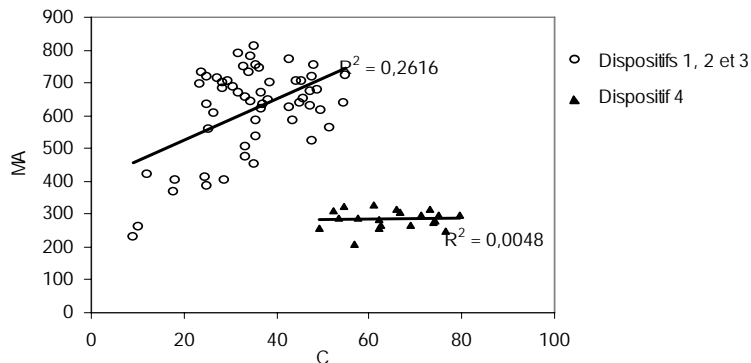
Figure 1-3 : Relations entre teneurs en MA (g.kg -1 sol) et la teneur en C (g.kg -1 sol) du sol sur les dispositifs d'Andranomanelatra, Bemasoandro et Ibity (Dispositifs 1, 2 et 3) et le dispositif de Betafo (Dispositif 4).
