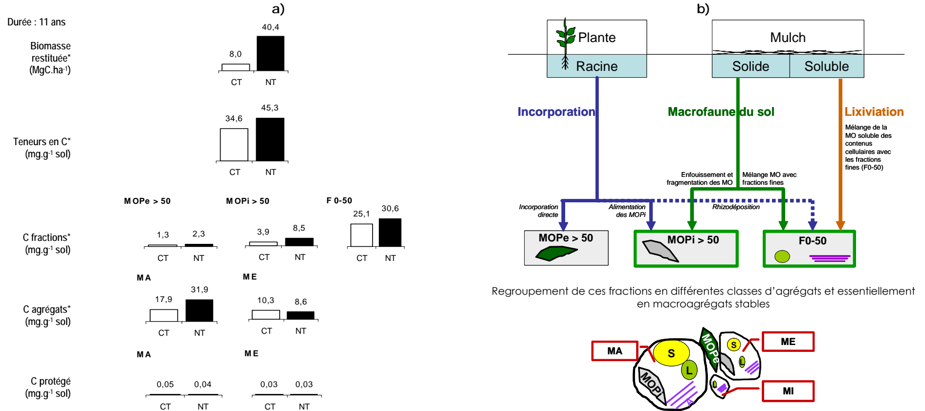
Figure 5-2 : Synthèse des résultats obtenus sur le système NT m/s et système CT m/s pour la couche de 0-5 cm de profondeur, Andranomanelatra. (a), et schéma explicatif des agents et processus pouvant être mis en jeu lors du stockage de C sous SCV (b).
