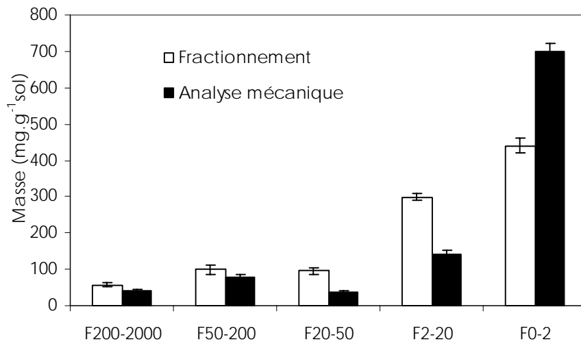
Figure 3-3 : Comparaison des masses moyennes des fractions issues du fractionnement granulométrique et de l'analyse mécanique pour l'ensemble des échantillons traités (moyenne \pm écart-type).
