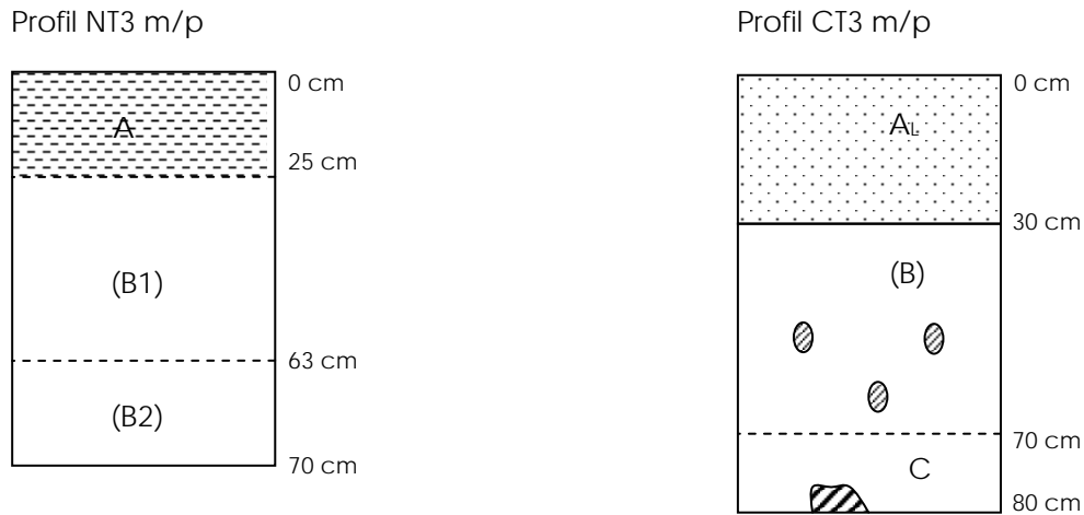
Figure 1-5 : Profils pédologiques observés sur le dispositif 3 (Ibity).
