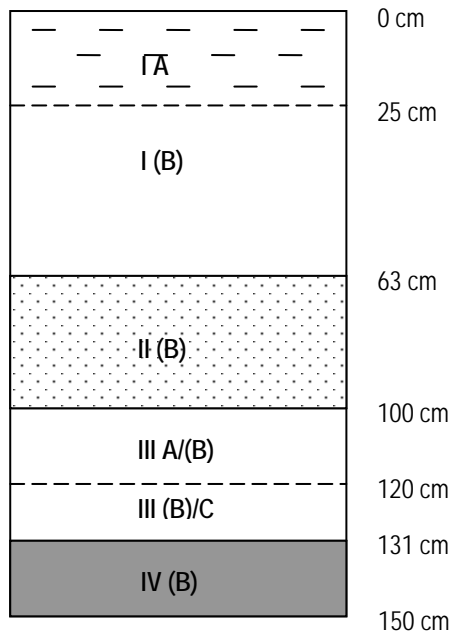
Figure 1-4 : Profils pédologiques observés sur le dispositif 2 (Bemasoandro).
