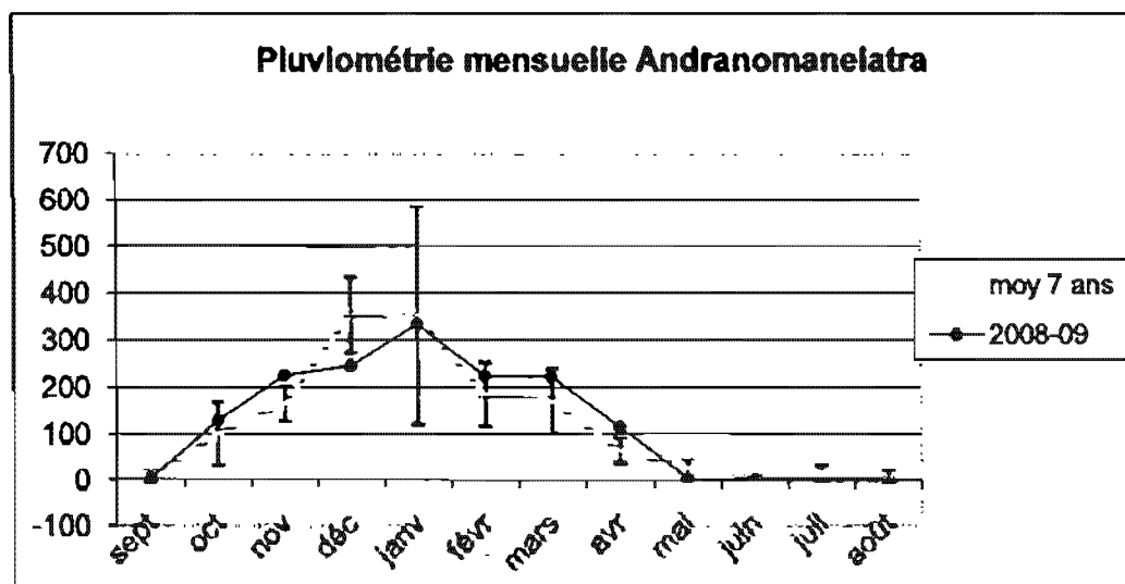
Figure n°01 : Pluviométrie mensuelle d'Andranomanelatra
