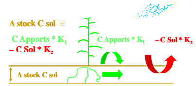
Fig.1. Modèle Hémin-Dupuis: C_t = C_0 * e^{-k_2 t} + k_1 / k_2 * A * (1 - e^{-k_2 t}) C t = stock C à un temps t C 0 = stock de départ k 2 = coefficient de minéralisation A = quantité C apporté k 1 = coefficient d'humification
